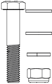
09TOR08 TORNILLERÍA PARA ASPAS 12X 01TINX101 TORNILLO 0.312" X 2.000" 24X 01TOR042 RONDANA PLANA 0.312" x 0.625" 12X 01TOR043 RONDANA DE PRESIÓN 0.312" X 0.625" 12X 01TOR044 TUERCA DE SEGURIDAD 0.312"
