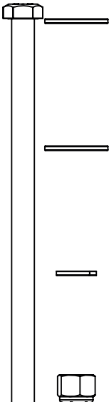
09TOR07 TORNILLERÍA PARA MONTAR XTRACTOR 8X 09TOR071 TORNILLO 0.500" X 8" 16X 01TOR012 RONDANA PLANA 0.500" 8X 01TOR013 RONDANA DE PRESIÓN 0.500" 8X 01TOR014 TUERCA DE SEGURIDAD 0.500"
